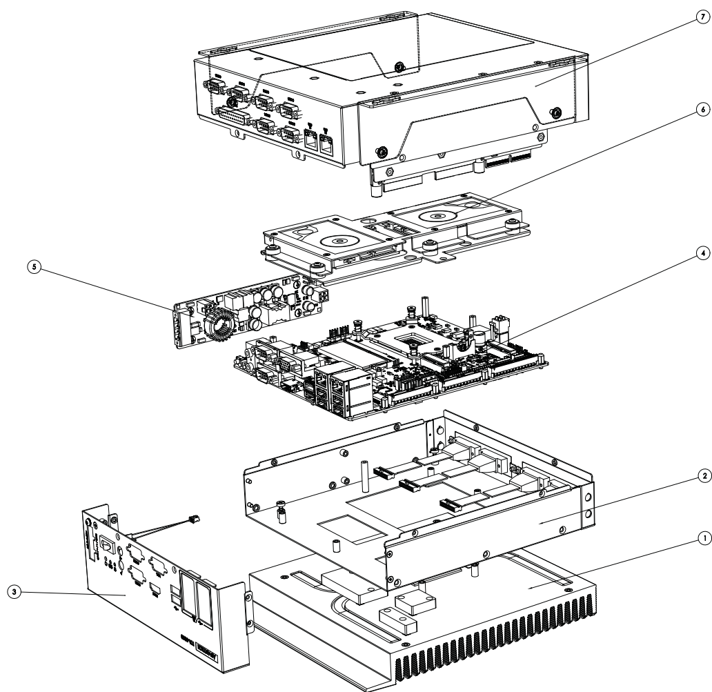
图 1.2: ITA-3650E 分解圖
