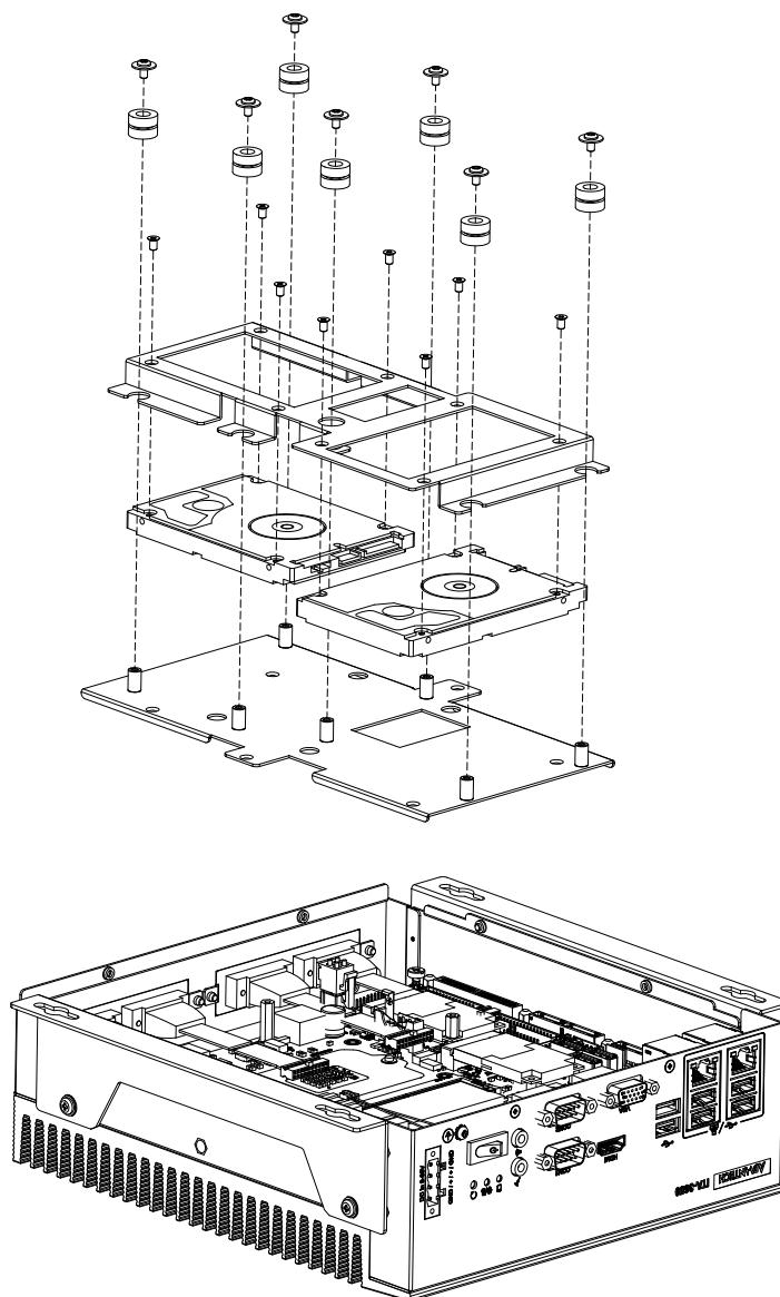
图 3.3：安装硬盘模块
