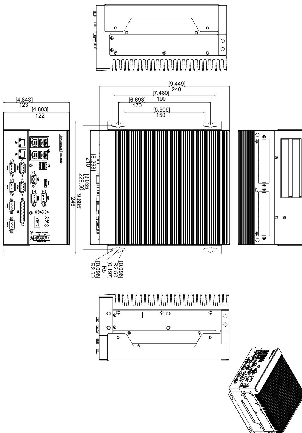
图 1.1: ITA-3650E 產品尺寸
