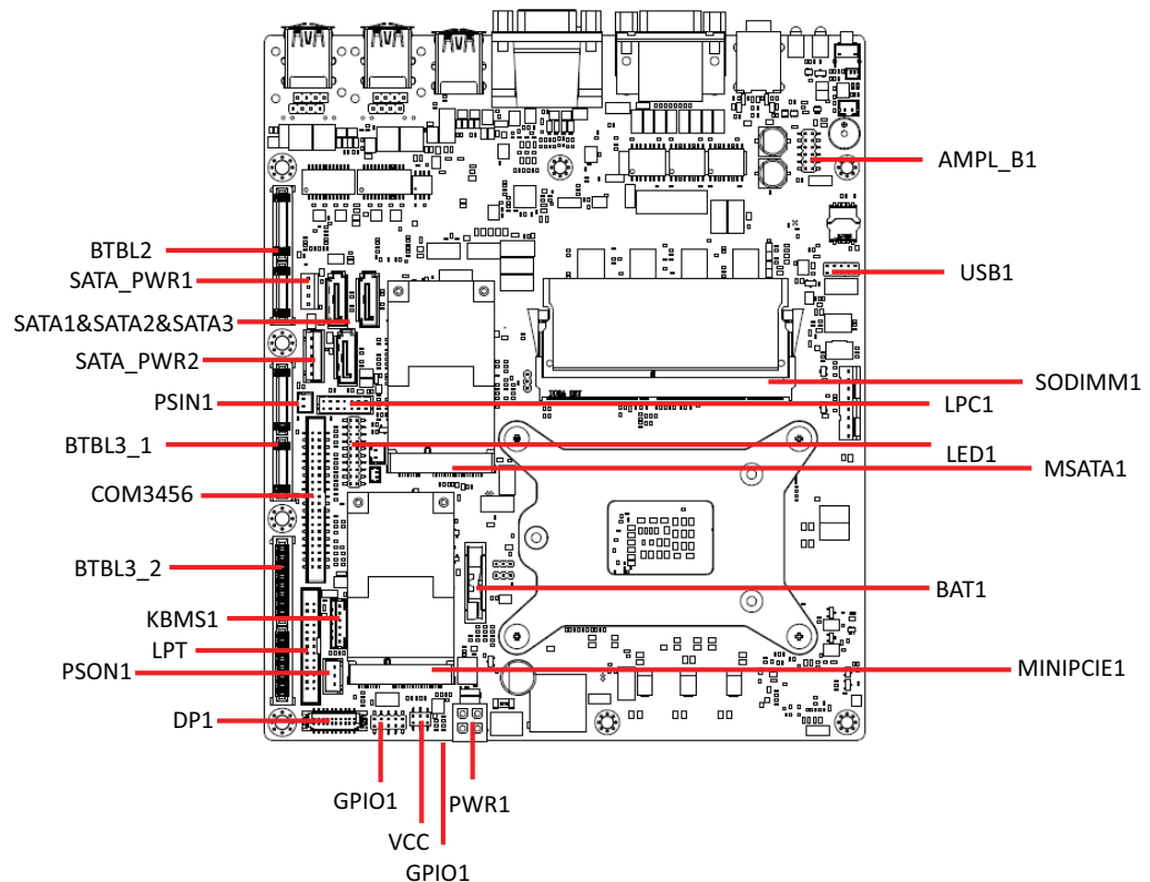
圖 2.2：主機板介面及跳線位置圖
