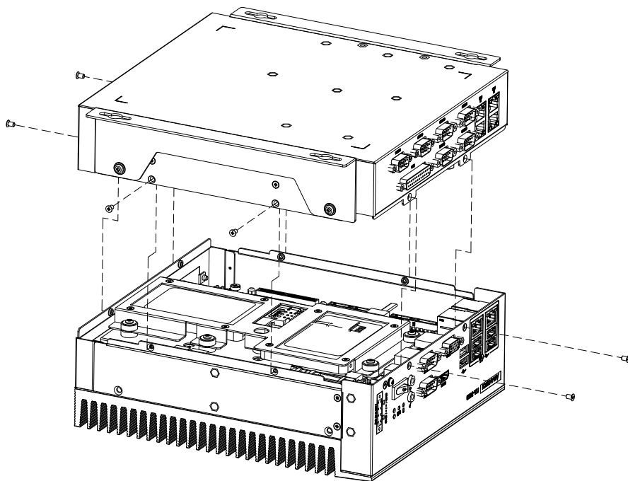
图 3.6：安裝模組
