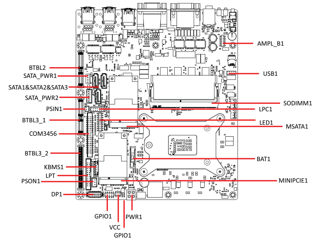
图 2.2：主板接口及跳线位置图
