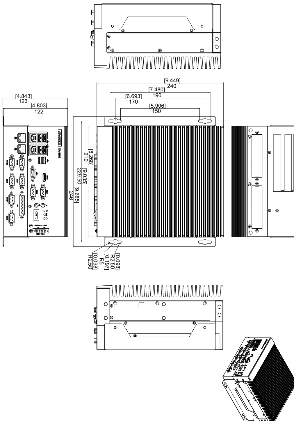
图 1.1: ITA-3650E 产品尺寸
