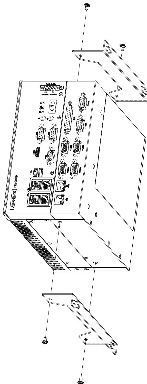
图 3.5: 安裝腳架
