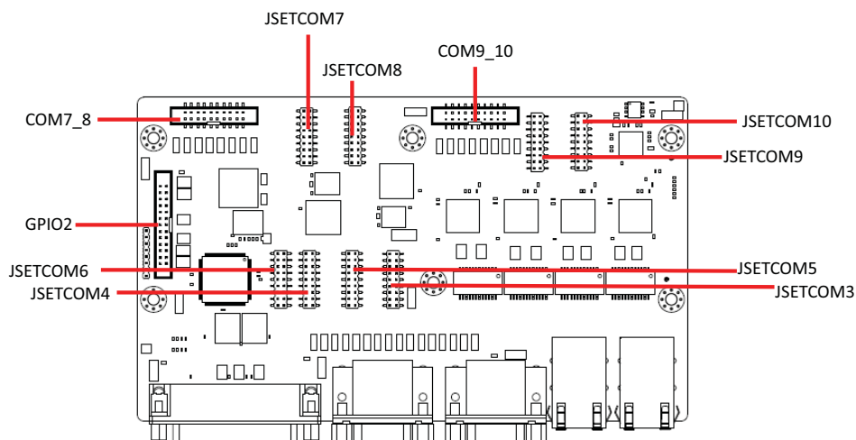
图 2.3: 扩展 I/O 板接口及跳线位置图
