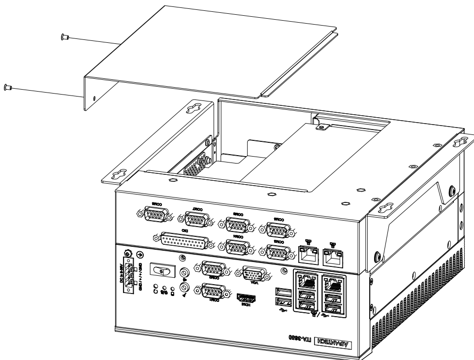
图 3.4：安装上盖
