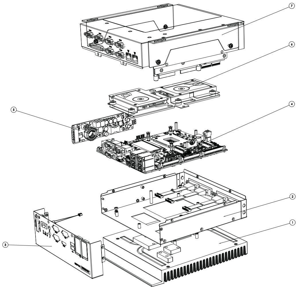
图 1.2: ITA-3650E 分解图
