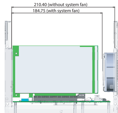
4-slot i-Module
