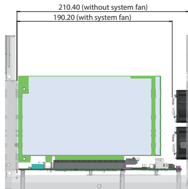
2-slot i-Module
