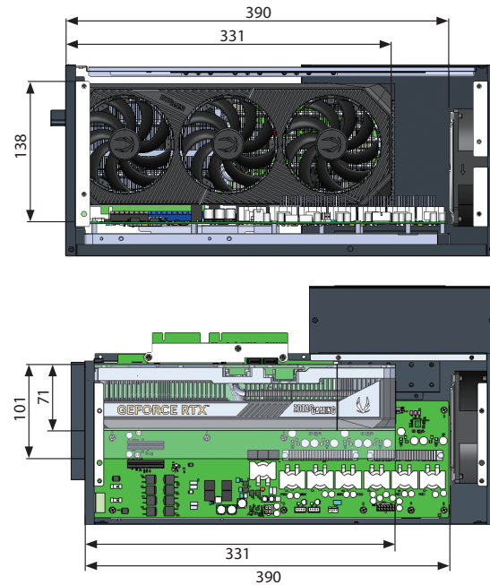
MIC-78G30 GPU Dimension Guide
